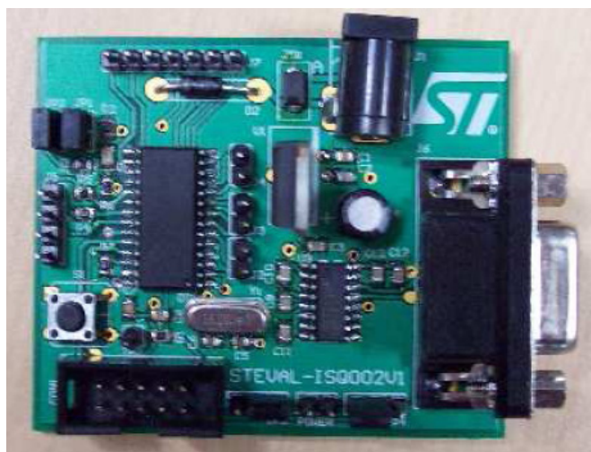
Figure 29. STEVAL-ISQ002V1
